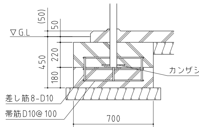
A-A' 断面 1/20
